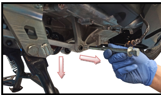
Sfilare la vite indicata ed abbassare l'ammortizzatore. Remove the screw as shown and lower the shock absorber
