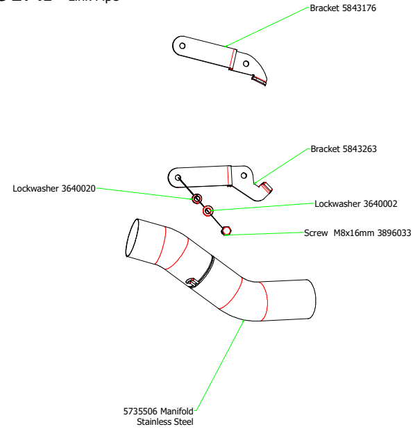
71451MI Link Pipe
